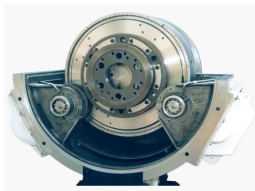
行星齿轮箱
